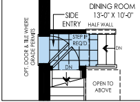
OPT. SIDE DOOR ENTRY
